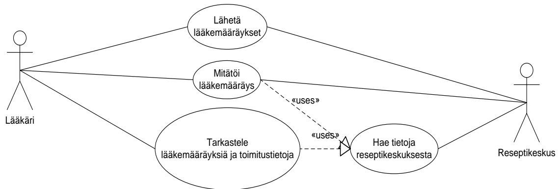
Kuva 8, Esimerkki käyttötapauskuvauksesta
