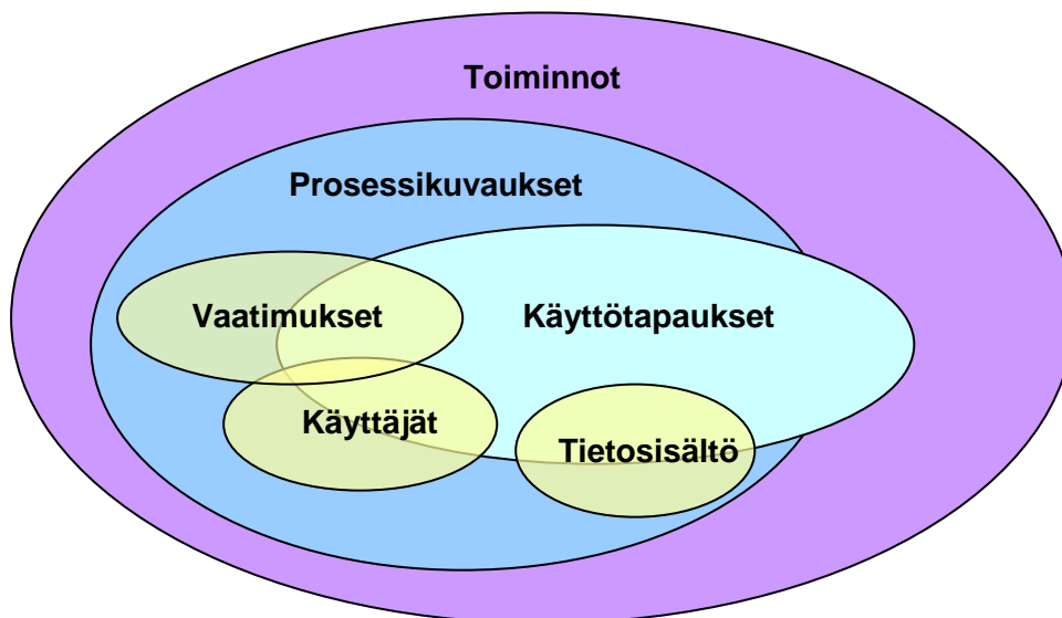
Kuva 7, Vaatimusmäärittelydokumentaation sisältö
