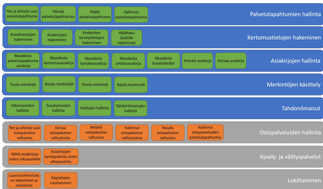
Kuva 2.2. Toiminnallisten vaatimusten jäsenyys.
