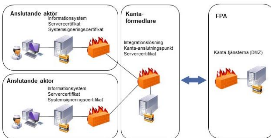
Figur 7: Anslutning via en anslutningspunkt som administreras av en Kanta-förmedlare
