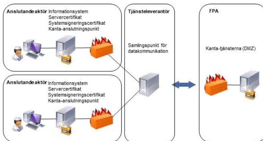
Figur 9: Anslutning med hjälp av samlingspunkt för datakommunikation
